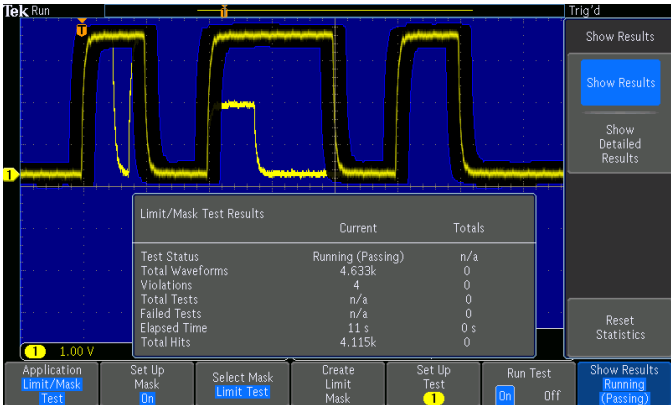
골든 파형에서 생성된 마스크를 실시간 신호와 비교한 한계 테스트. 테스트에 대한 통계 정보를 보여주는 결과가 표시됩니다.
