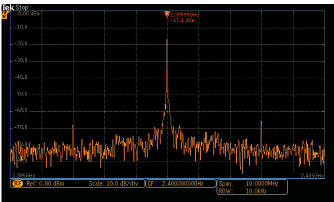
MDO3000 주파수 영역 디스플레이
